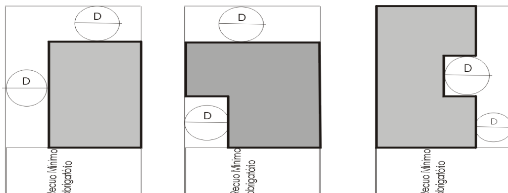
1 - ÁREAS ABERTAS E SEMI-ABERTAS PARA ILUMINAÇÃO E VENTILAÇÃO Dimensões mínimas das Seções Horizontais
